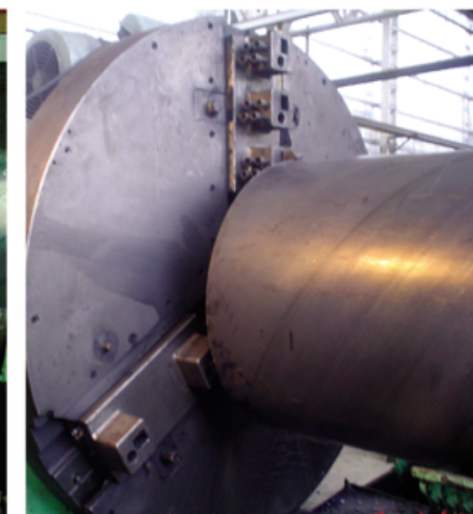
End Beveling
